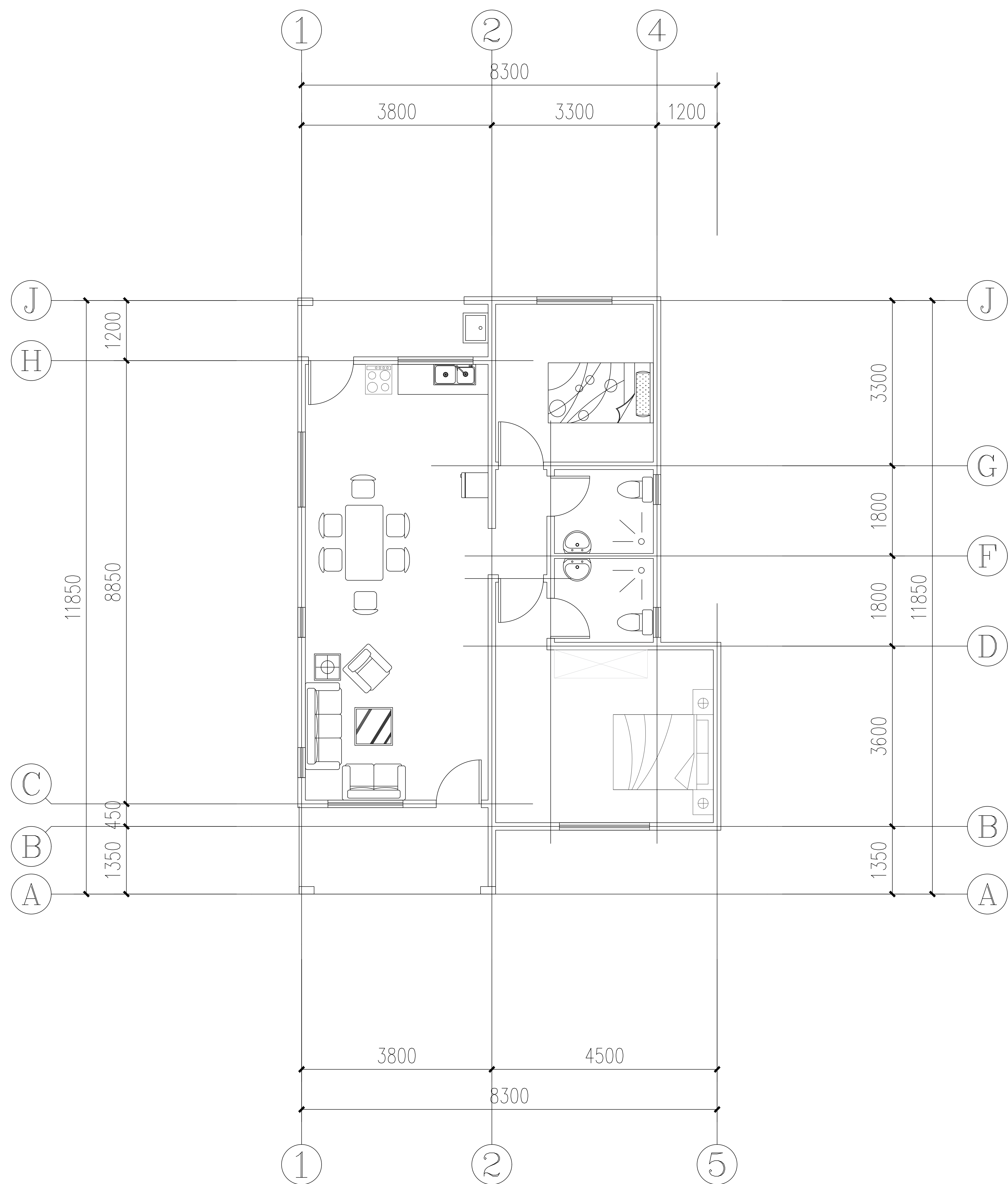
T2户型平面布置图 1:100
